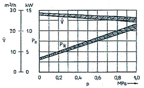
Baugröße 25
