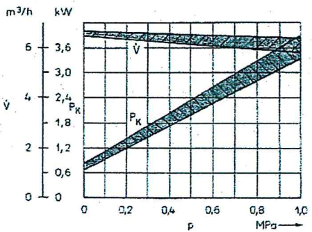
Baugröße 6,3
