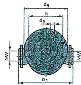
Baugrößen 40 bis 63
