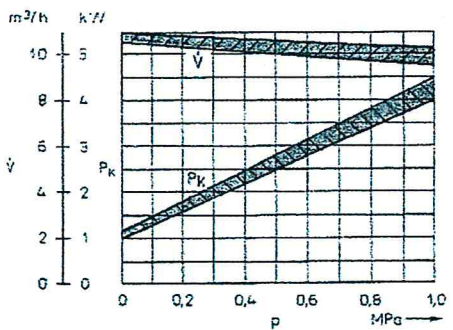
Baugröße 10
