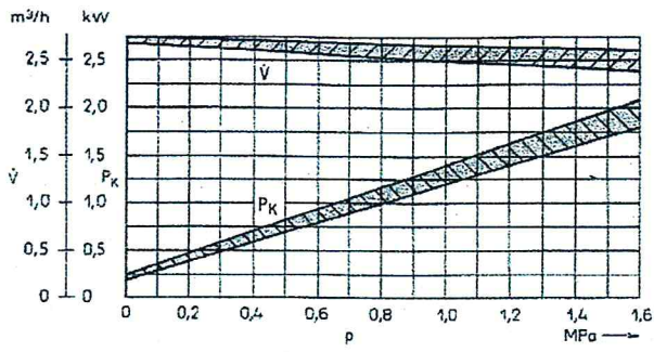
Baugröße 2,5
