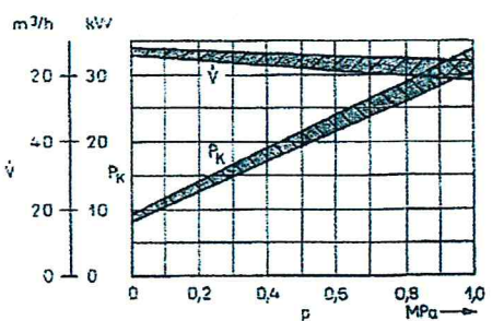
Baugröße 63
